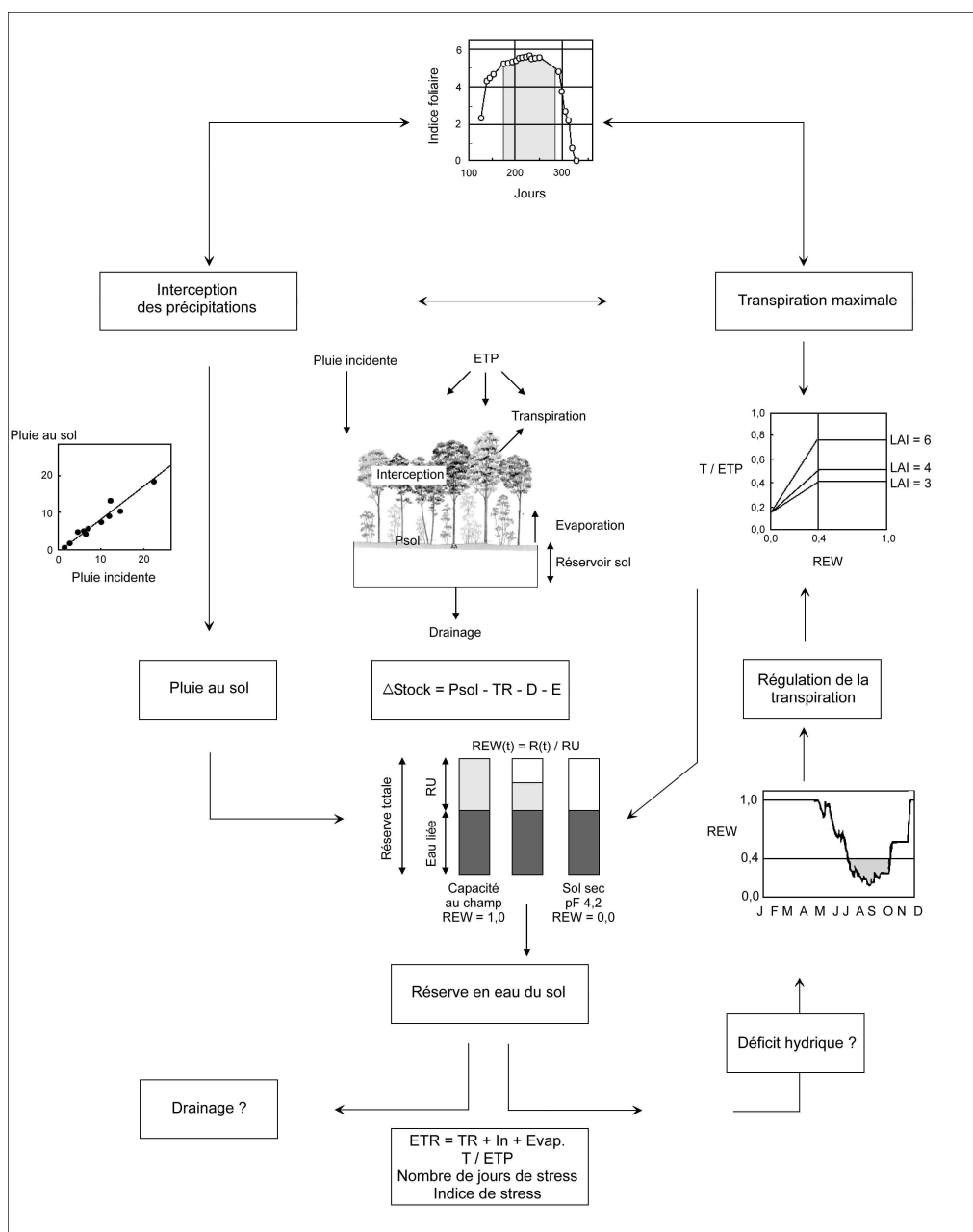
Figure 30 : Schéma général du modèle de bilan hydrique journalier. D'après Granier et al. , 1995.
