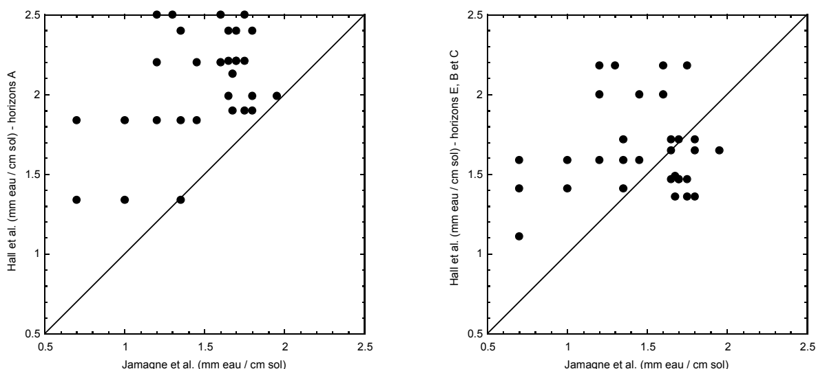
Figure 24 : Comparaison des quantités d'eau utile des études de Jamagne et al. (1977) et Hall et al. (1977).
