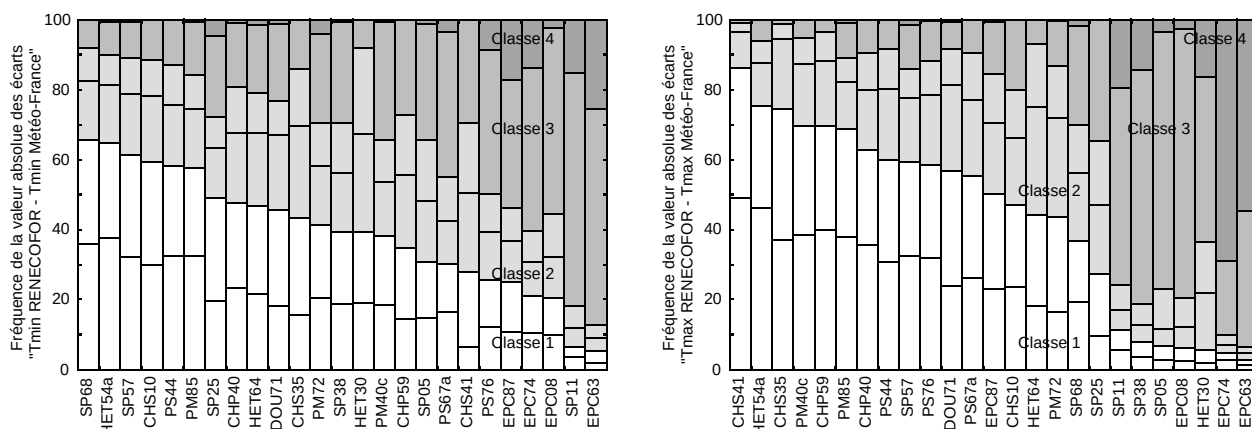
Figure 6 : Fréquence de la valeur absolue des écarts entre les températures journalières mesurées sur les placettes RENECOFOR et les stations Météo-France. A gauche, cas des températures minimales ; à droite, cas des températures maximales. Classe 1 = [0-0,5°C] et [0,5-1°C] (même couleur), classe 2 = [1-1,5°C] et [1,5-2°C] (même couleur) ; classe 3 = [2-5°C] ; classe 4 = 5°C.
