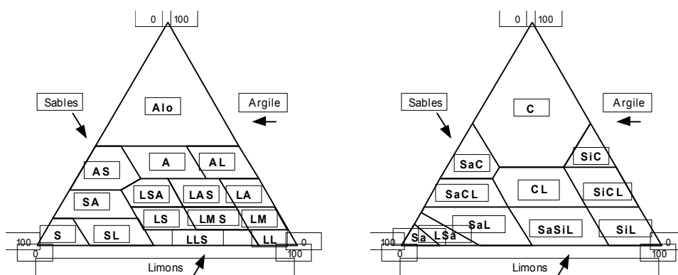
Figure 23 : Diagrammes de classification des textures : à gauche, Service de Cartographie des Sols de l'Aisne (Jamagne, 1967, in Baize, 2000) ; à droite, Soil Survey of England and Wales (Hall et al. , 1977) - (la limite limon / sable est ici à 60 µm et non pas à 50 µm comme dans le système international).
