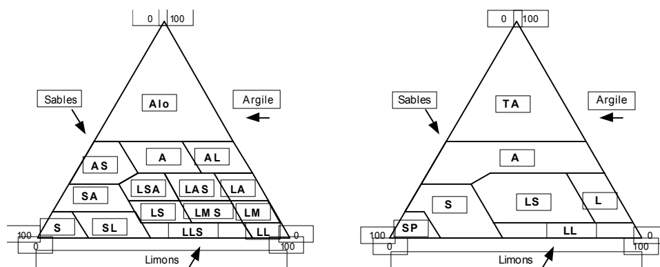
Figure 25 : Diagrammes de classification des textures : à gauche, Service de Cartographie des Sols de l'Aisne (Jamagne, 1967, in Baize, 2000) ; à droite, utilisé par Chapelier et al. (1999) – (cf.texte)
